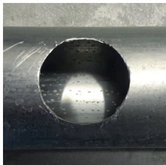
Před aplikací zdrsňte a odmaštěte plochu. (Pro odmaštění použijte 123 Fluid Extra)
