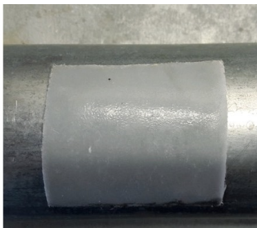
Přitiskněte bandáž a nechte vytvdřit UV zářením. (Slunce - 50 min. / UV lampa - 5 min.)
